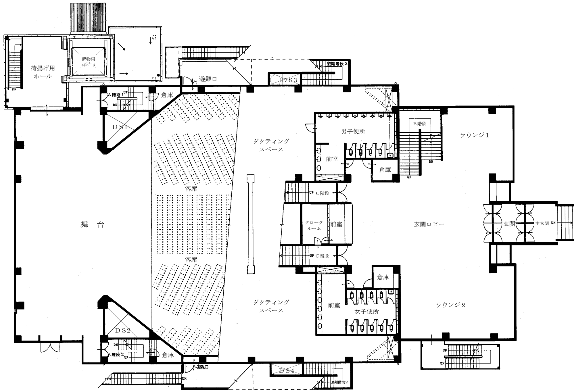
2階平面図
