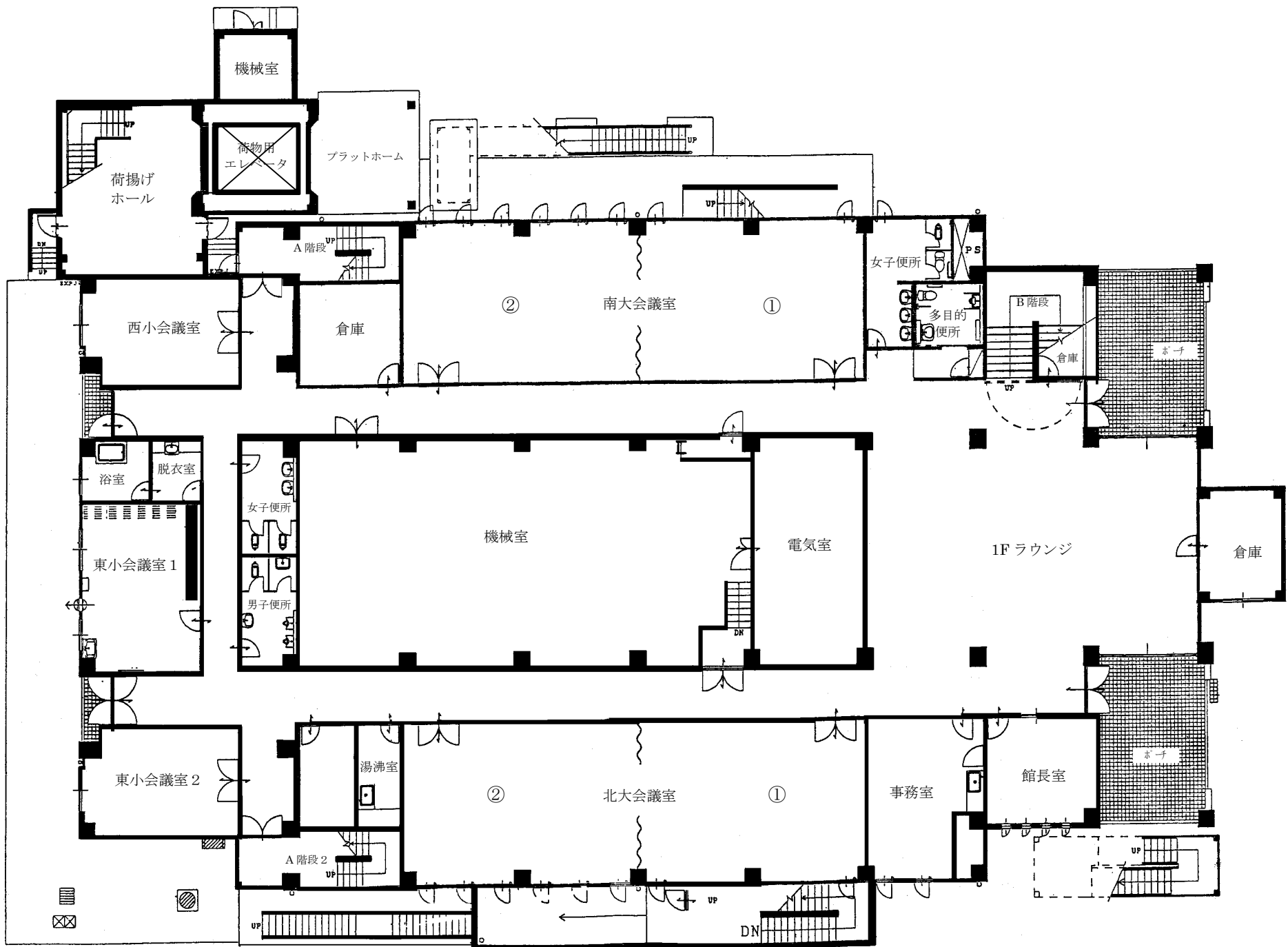
1 階平面図
